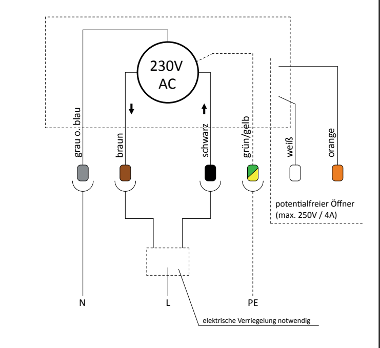
Schaltbild zeigt: JM-B 500 - 500 - LS
