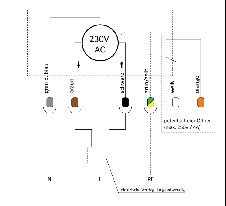
Schaltbild zeigt: JM B 500 - 300 - LS
